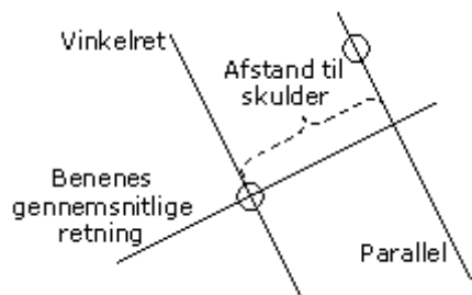
Figur 56 – Afstanden fra benenes gennemsnitlige placering til skulderen i løberetningen.
