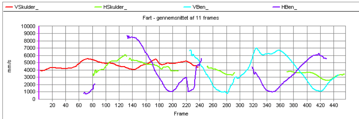
Figur 53 – Fart som gennemsnit af 11 frames.
