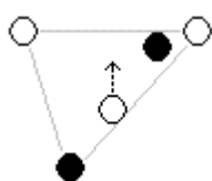
Figur 34 – Ved acceleration læner man sig forover.
