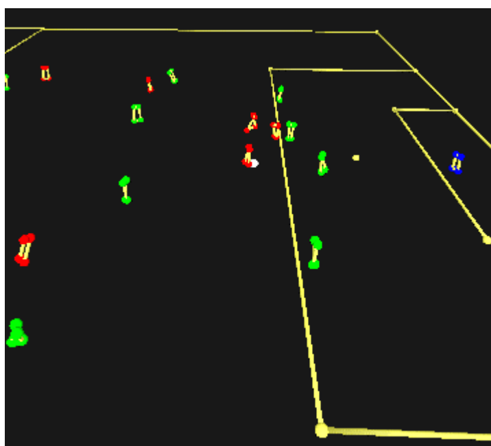
Figur 58 – Øjeblikbillede fra scenario afspillet i Qualisys Track Manager.
