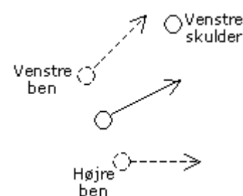
Figur 55 – Føddernes placering og retning samt skulderens placering.
