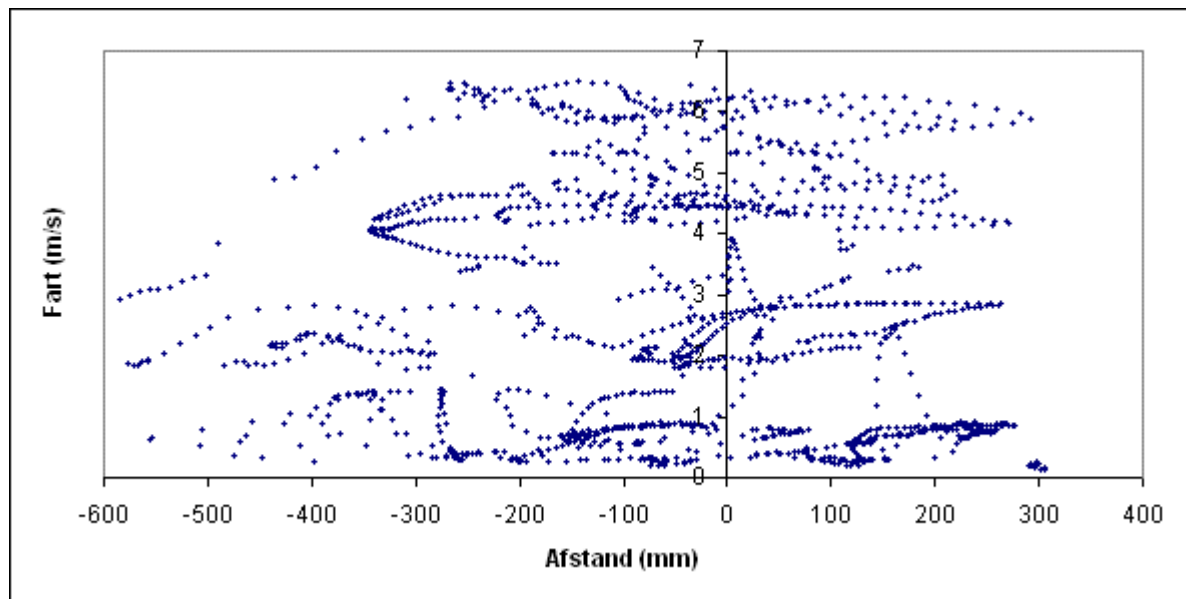
Figur 31 – Afstand fra forreste ben i løberetningen til skulderen.
