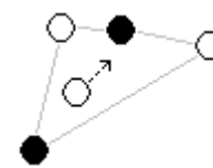
Figur 33 – Ved retningsskift læner man sig til siden.
